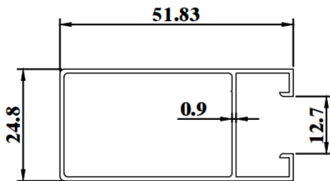
ESD179A WEIGHT : 0.400 KG/M AP : 206.03mm
