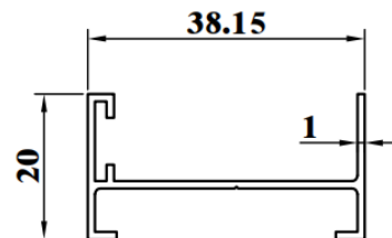
ESD169C WEIGHT : 0.243 KG/M AP : 178.68mm
