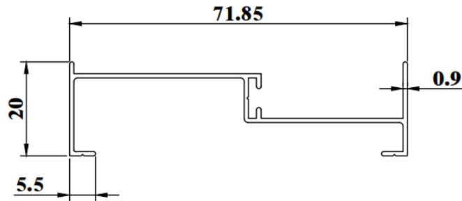
ESD170AB WEIGHT : 0.332 KG/M AP : 270.74mm
