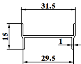
ESD177C WEIGHT : 0.159 KG/M AP : 117.82mm
