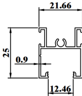
ESD173A WEIGHT : 0.254 KG/M AP : 202.56mm
