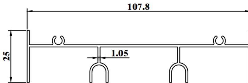
ESD170AB WEIGHT : 0.332 KG/M AP : 270.74mm
