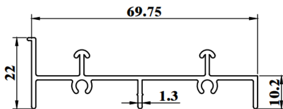
ESD175H WEIGHT : 0.533 KG/M AP : 295.46mm
