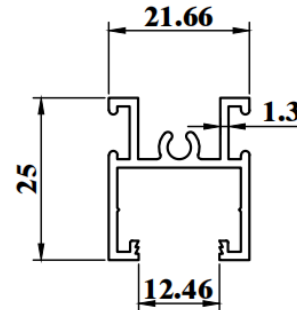
ESD173H WEIGHT : 0.347 KG/M AP : 198.89mm
