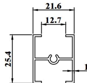
ESD182C WEIGHT : 0.245 KG/M AP : 182.11mm
