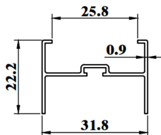
ESD184A WEIGHT : 0.208 KG/M AP : 170.02mm
