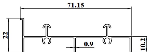
ESD175A WEIGHT : 0.383 KG/M AP : 299.93mm
