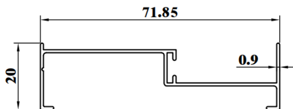
ESD170A WEIGHT : 0.326 KG/M AP : 255.99mm
