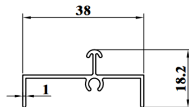
ESD176C WEIGHT : 0.211 KG/M AP : 153.09mm
