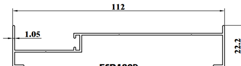
ESD180D WEIGHT : 0.511 KG/M AP : 359.66mm
