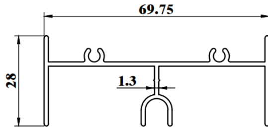
ESD171H WEIGHT : 0.608 KG/M AP : 339.48mm
