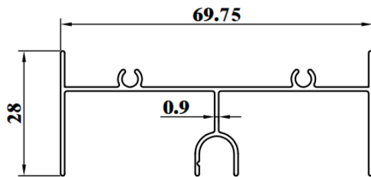
ESD171A WEIGHT : 0.431 KG/M AP : 340.87mm
