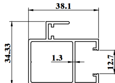
ESD174H WEIGHT : 0.553 KG/M AP : 226.56mm
