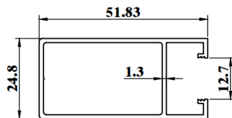
ESD179H WEIGHT : 0.565 KG/M AP : 205.82mm
